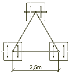
Stomme till skyltställ typ 3 Plan sedd uppifrån
