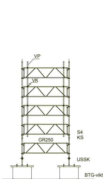
Stomme till skyltställ typ 3 Med höjd 6,0m
